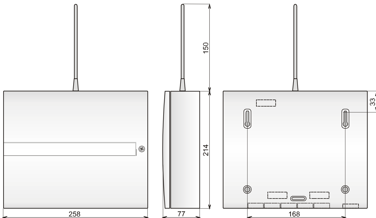
Wymiary
