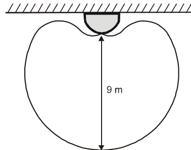
Pole detekcji czujnika zbitcia szkła
