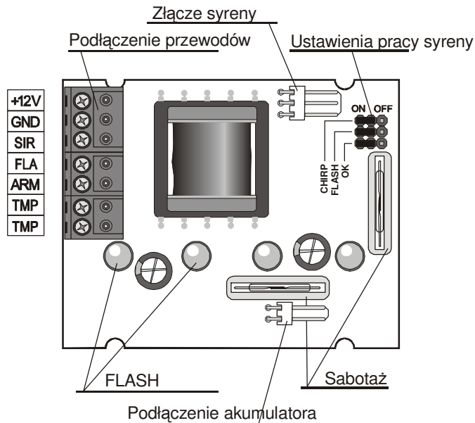
Rysunek 1. Płyta główna syreny
